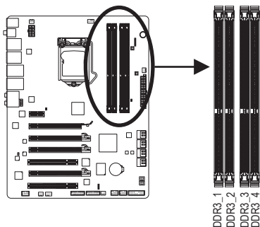
▶▶ Двухканальный режим работы ОЗУ: таблица конфигурации
