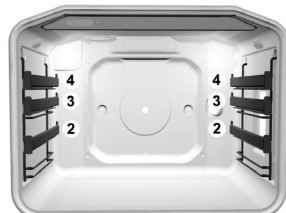
телескопические направляющие
