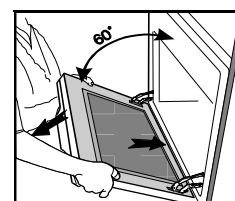
2 Петля дверцы при снятии
