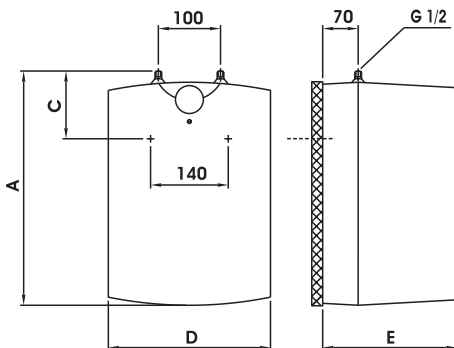
Модел под умиваоницом
