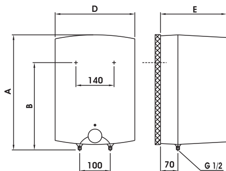
Модел над умиваоницом
