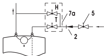
Uitvoering voor montage onder de wastafel
