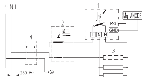
Schéma du couplage électrique
