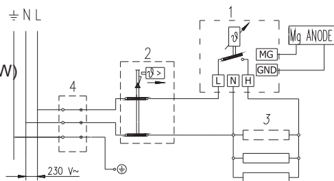
Schema legăturii electrice
