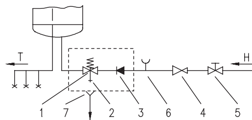
Sistema fechado (de pressão)
