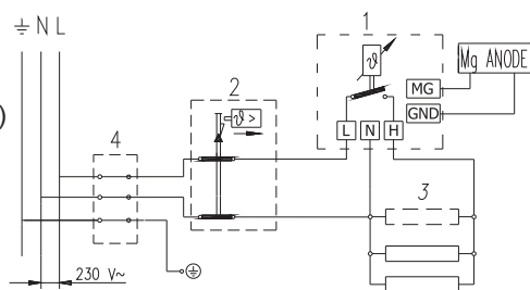
Schéma elektrického zapojenia
