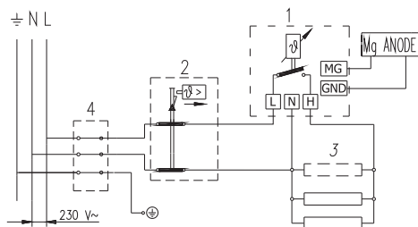
Esquema de la conexión eléctrica
