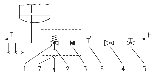
Das Drucksystem
