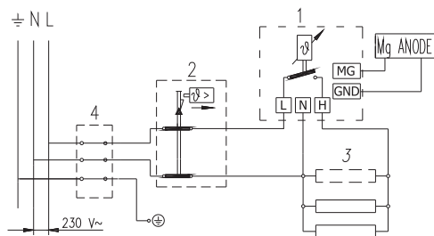
Skema e lidhjes elektrike
