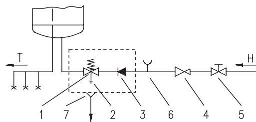
Затворен систем (со притисок)
