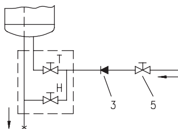
Sistema aberto (sem pressão)
