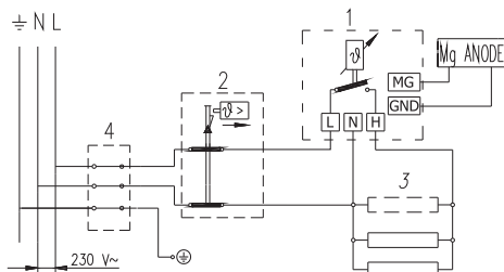
Електросхема
