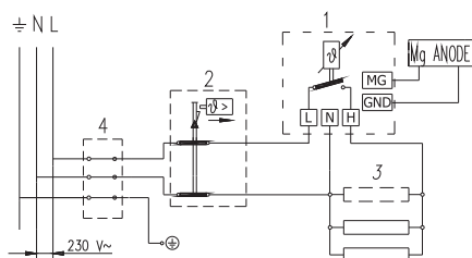
instalação elétrica
