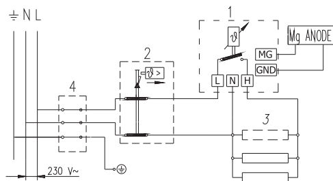
Schema van de elektrische verbinding
