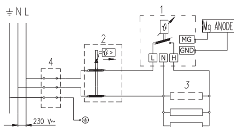
Shema električne vezave
