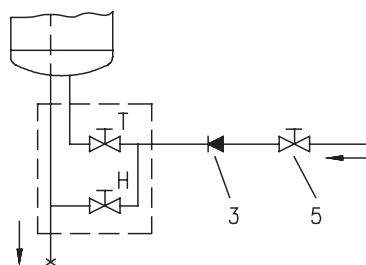
Das Durchflußsystem
