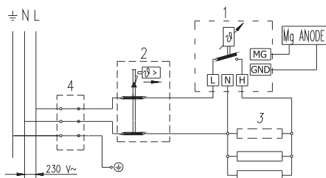
Шема на електрично поврзување
