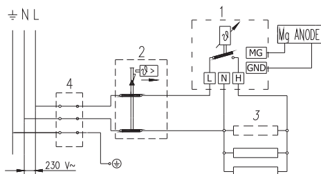
Das Schaltungsschema des Elektroanschlusse
