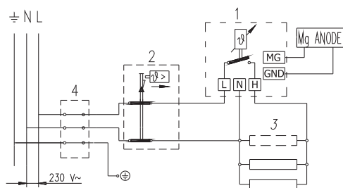
Электросхема
