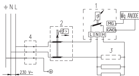
Električna spojna shema
