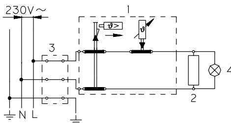
Электросхема
