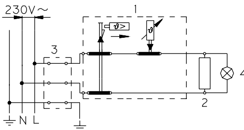
Schema električne vezave
