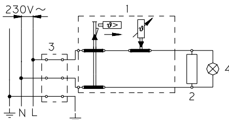
Elektroschema
