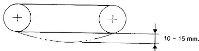
Tension de la chenille en caoutchouc.
