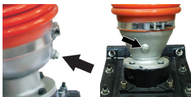
Маслосливное отверстие
