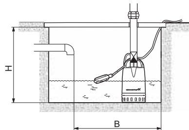
Рис. 3 Минимальные габаритные размеры
