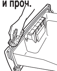
Паз для крепления прокладки вакуумного отделения
