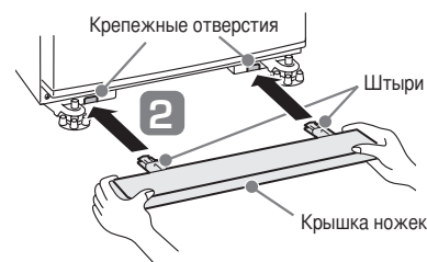
Крепежные отверстия
