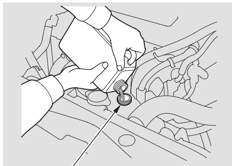
ЗАЛИВНАЯ ГОРЛОВИНА РАДИАТОРА
