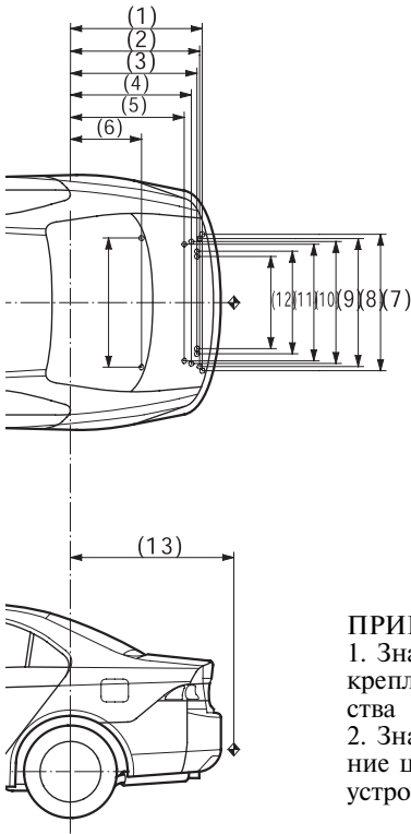
Расположение точек крепления тягово-сцепного устройства для буксировки прицепа
