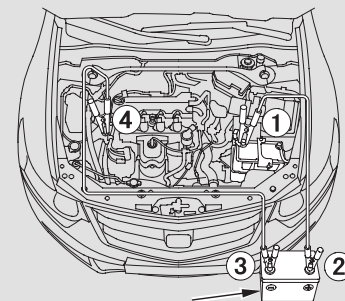
ВНЕШНЯЯ АККУМУЛЯТОРНАЯ БАТАРЕЯ
