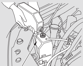
РАСШИРИТЕЛЬНЫЙ БАЧОК
