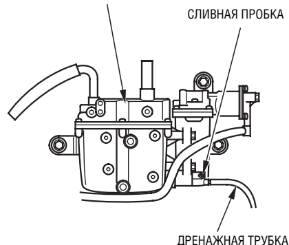
СЕПАРАТОР ПАРОВ ТОПЛИВА
