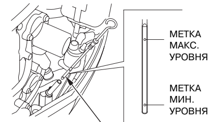
МАСЛЯНЫЙ ЩУП
