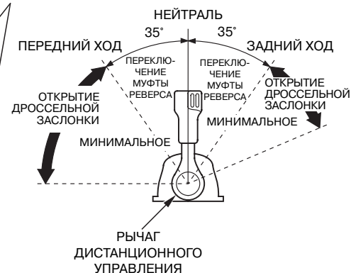
ЗАДНИЙ ХОД
