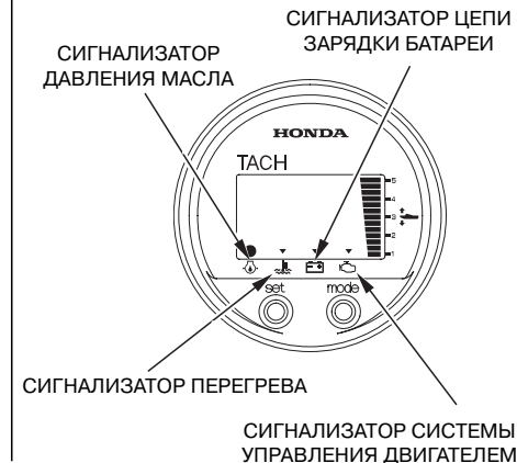
ЦИФРОВОЙ ТАХОМЕТР
