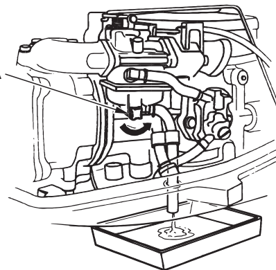
СЛИВНАЯ ПРОБКА
