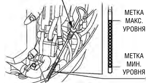
КОНТРОЛЬНЫЙ МАСЛЯНЫЙ ЩУП
