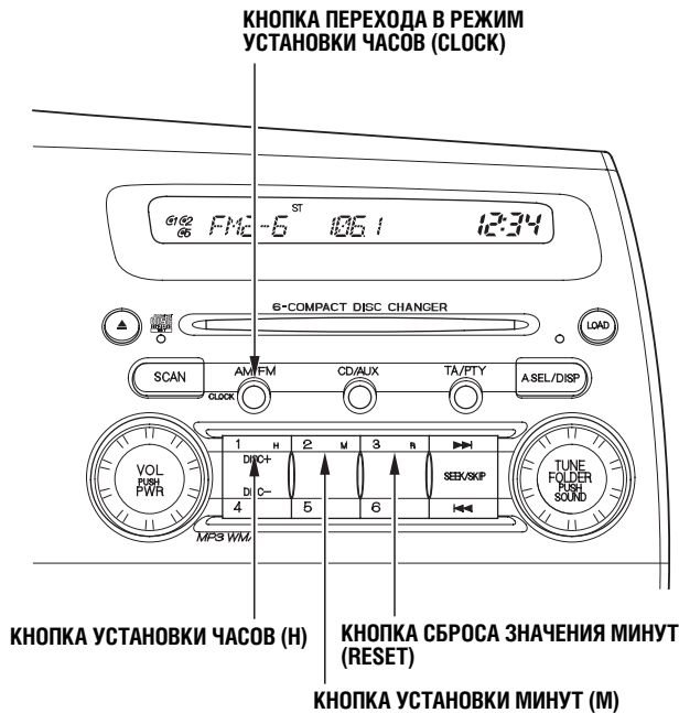
Аудиосистемы D, E, F и G
