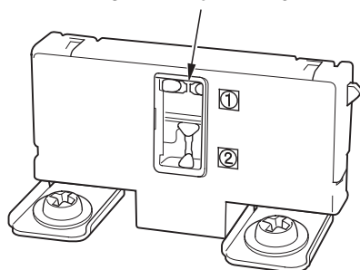
ПЕРЕГОРЕВШАЯ ПЛАВКАЯ ВСТАВКА
