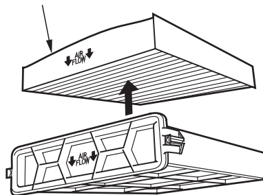
ФИЛЬТРУЮЩИЙ ЭЛЕМЕНТ
