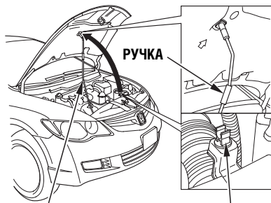
ДЕРЖАТЕЛЬ
