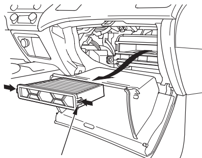
ФИКСАТОР
