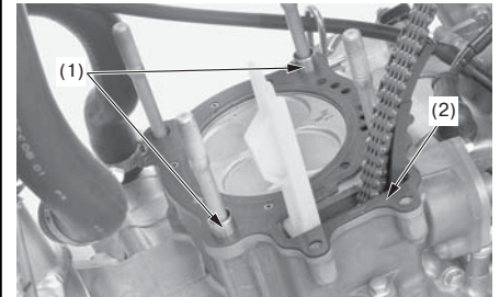
(1) установочные шпильки (2) прокладка головки цилиндра
