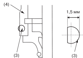
(3) изнашиваемая втулка
