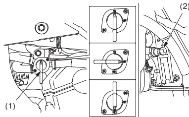
(1) топливный кран
