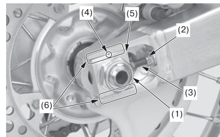
(1) гайка задней оси (4) установочная метка (2) контргайка (5) стопорная пластина (3) регулировочный болт (6) референтные метки
