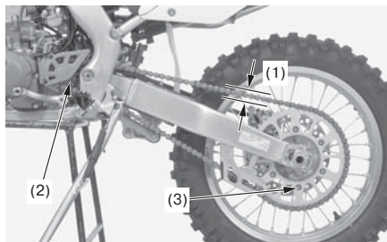
(1) прогиб приводной цепи (3) ведомая звездочка (2) ведущая звездочка
