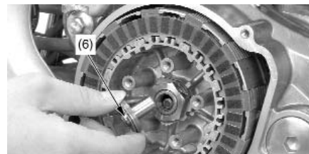
(6) механизм выключения сцепления в сборе
