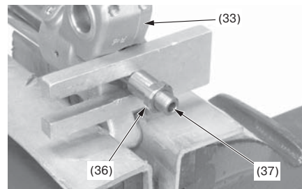
(33) держатель оси (36) контргайка
