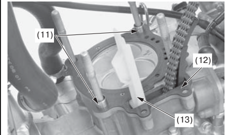
(11) установочные шпильки (12) прокладка головки цилиндра (13) направляющая цепи распредвала
