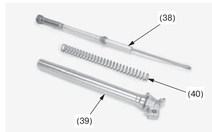
(38) узел демпфера вилки (39) узел вилки
