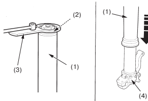
(1) внешняя труба (2) демпфер вилки (3) гаечный ключ (4) нижний торец внешней трубчатого наконечника
