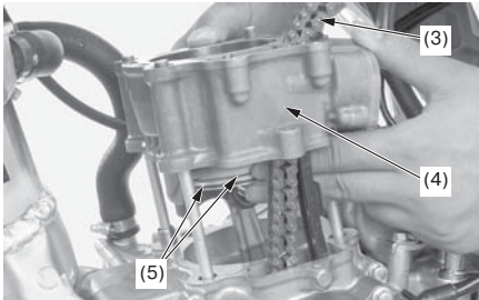
(3) цепь распредвала (4) цилиндр (5) поршневые кольца
