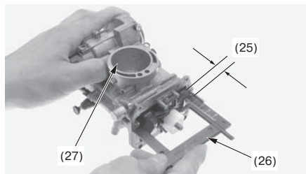
(25) верхнее положение поплавка (26) поплавковый уровень (27) впускное окно
