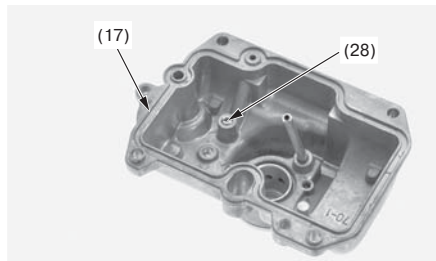
(17) поплавковая камера (28) обратный жиклер
