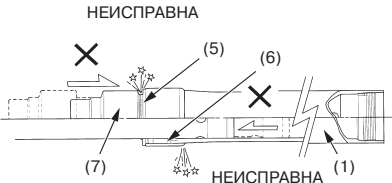
(1) внешняя труба (5) сальник (6) направляющая втулка (7) трубчатый наконечник
