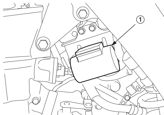
(1) конденсатор
