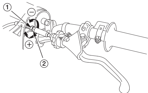
(1) контргайка (2) интегрированный регулятор (+) увеличить (–) уменьшить
