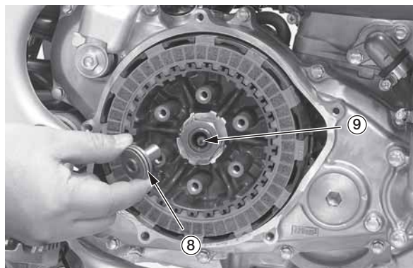
(8) толкатель сцепления (9) шток толкателя сцепления
