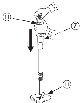
(7) воздушная/масляная камера (11) техническая салфетка
