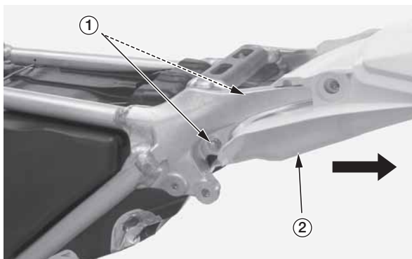
(1) болты заднего крыла (2) заднее крыло
