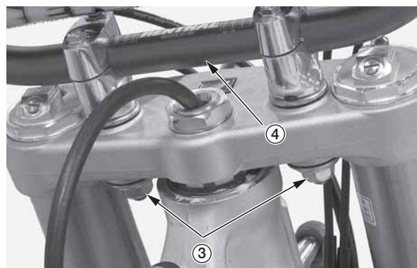
(3) нижние крепежные гайки руля, шайбы и установочные прокладки (4) руль
