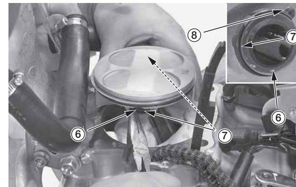
(6) поршневой палец (7) стопорные кольца поршневого пальца (новые) (8) вырезы на поршне
