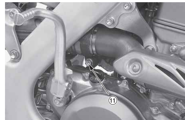
(11) болт хомута левого глушителя
