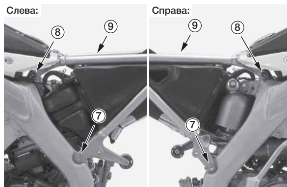
(7) Нижние болты подрамника (8) Верхние болты подрамника (9) Подрамник
