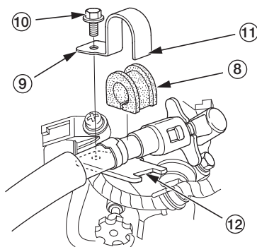
(8) Резиновая прокладка
