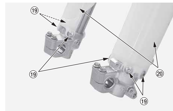
(19) болты защитных панелей вилки
