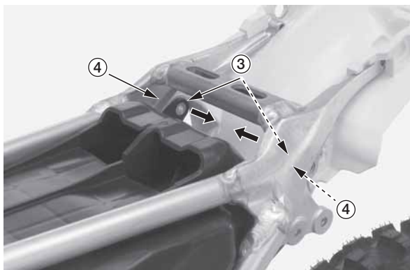
(3) корпус воздушного фильтра (4) подрамник
