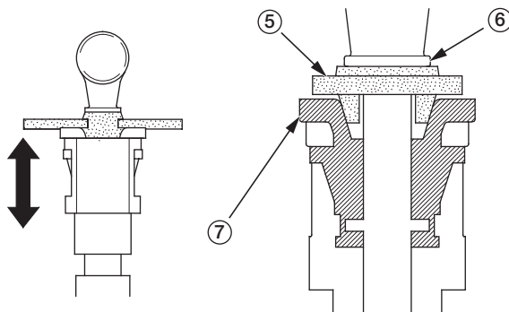
(5) резиновый соединитель (со стороны инжектора)
