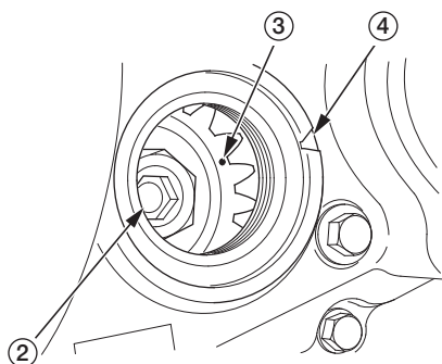
(2) болт первичной ведущей шестерни (3) центровочная отметка (4) контрольная отметка
