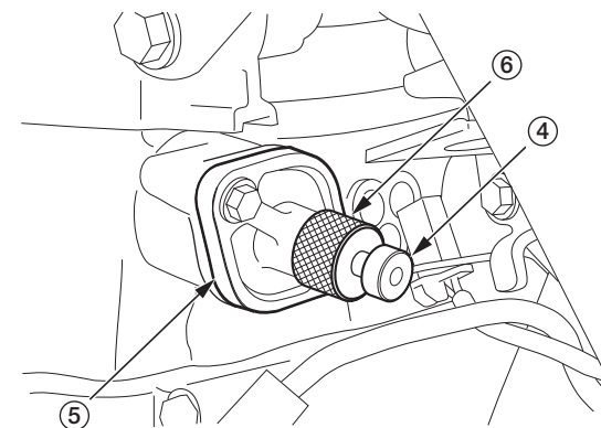
(4) стопорный натяжитель (5) ролик натяжения цепи распределительного вала (6) ручка
