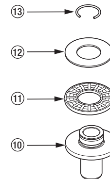
(10) толкатель сцепления (11) игольчатый подшипник (12) уплотнитель (13) фиксатор
