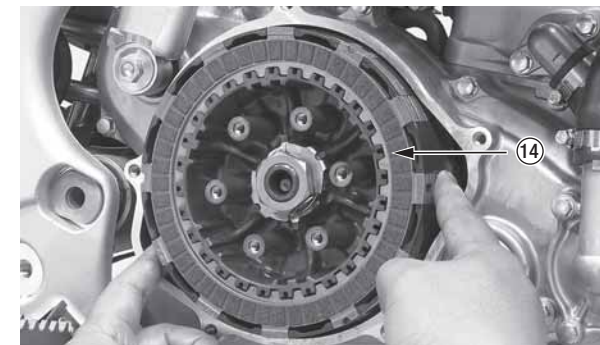
(14) фрикционные диски, гладкие диски, тарельчатая пружина, плоская шайба
