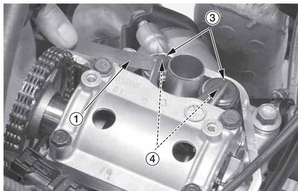
(1) щуп (3) коромысла выпускных клапанов (4) шайбы выпускных клапанов
