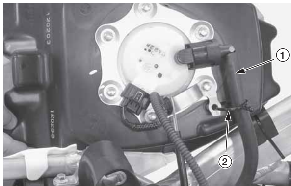
(1) топливопровод (2) хомут
