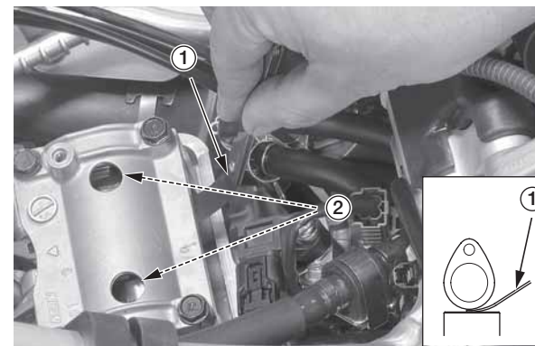
(1) щуп (2) толкатели клапанов и контуры кулачков клапанов
