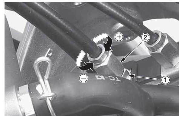
(1) контргайка
