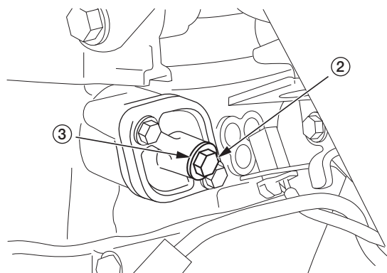
(2) болт кожуха (3) герметичная прокладка
