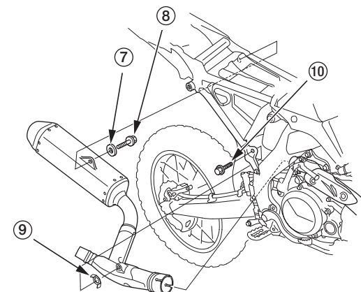
(7) шайба «В» (8) крепежный болт «В» левого глушителя (9) шайба «А» (10) крепежный болт «А» левого глушителя
