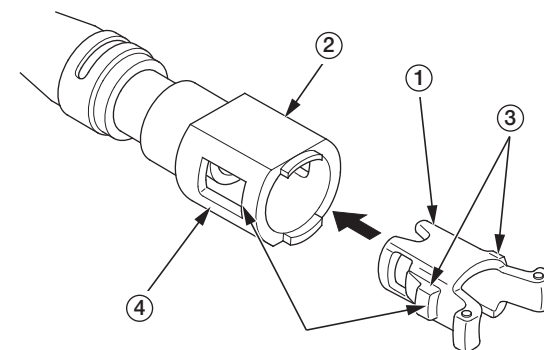
(1) держатель (новый)
