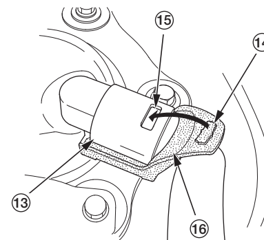
(13) соединение топливпровода
