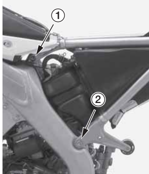
(1) верхние болты подрамника (2) нижние болты подрамника
