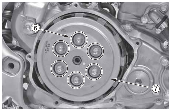
(6) пружины и болты сцепления (7) прижимной диск сцепления
