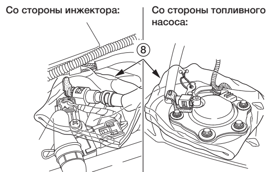
(8) техническая салфетка
