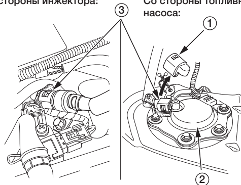
(1) крышка соединения топливопровода
