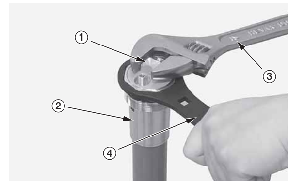
(1) узел наконечника вилки (2) демпфер вилки (3) разводной ключ (4) накидной ключ
