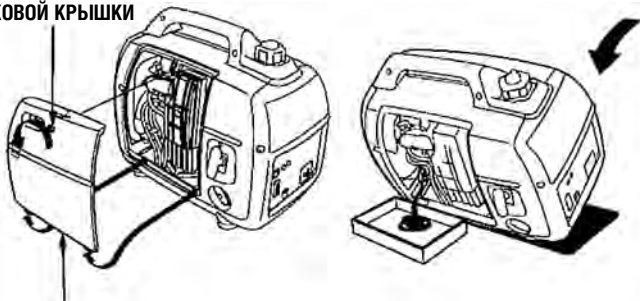
БОКОВАЯ КРЫШКА
