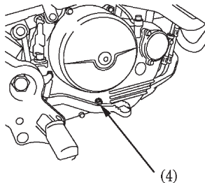
(4) Болт отверстия для проверки уровня масла
