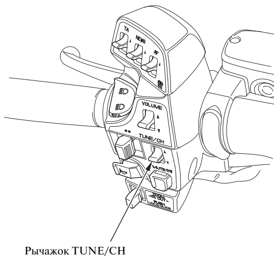
Рычажок TUNE/CH
