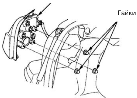
Задний указатель поворота в сборе
