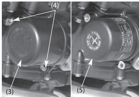
(3) Крышка масляного фильтра (4) Болты (5) Масляный фильтр
