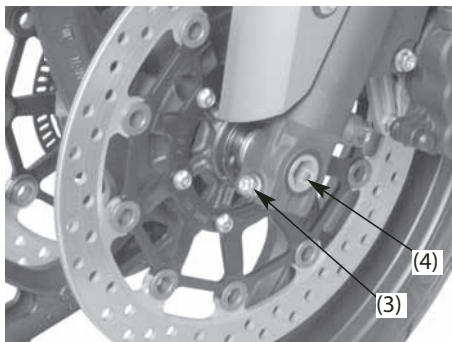
(3) Стяжной болт оси (4) Передняя ось
