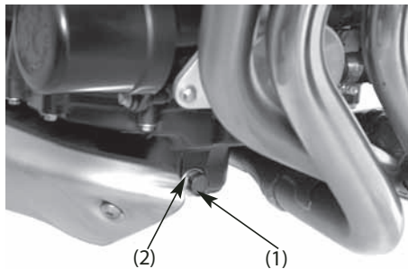
(1) Сливная пробка (2) Уплотнительная шайба
