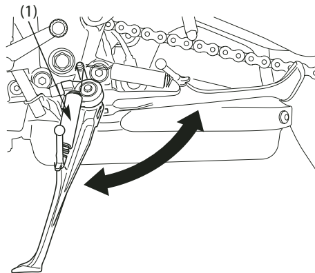
(1) Пружина бокового упора
