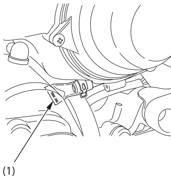
(1) Дренажная трубка
