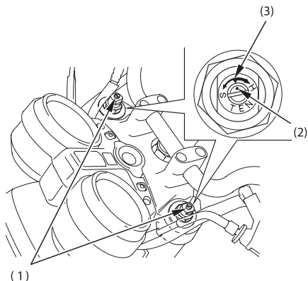
(1) Регулятор отбоя
