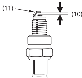
(10) Зазор (11) Боковой электрод
