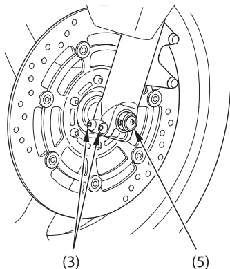
(3) Осевые болты (5) Вал передней оси
