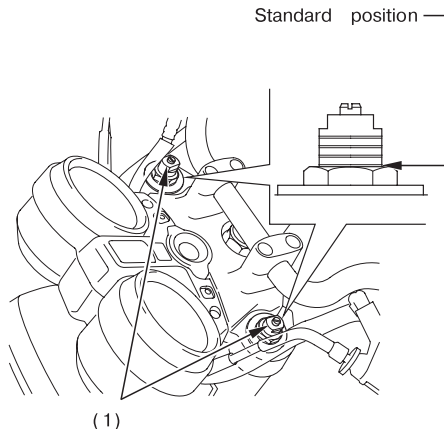
(1) Регулятор предварительной накрутки
