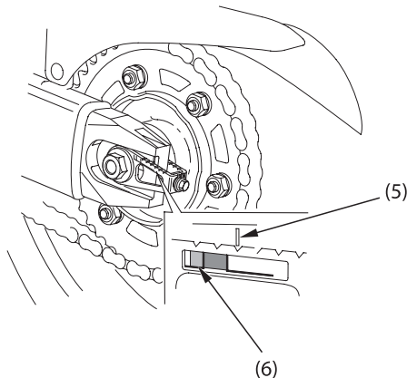
(5) Метка
