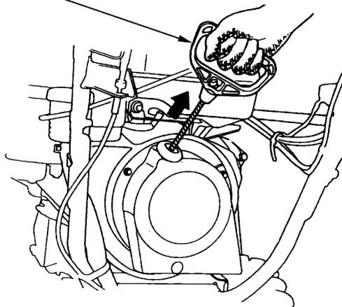
РУКОЯТКА СТАРТЕРА
