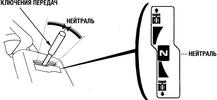
РЫЧАГ ПЕРЕКЛЮЧЕНИЯ ПЕРЕДАЧ
