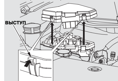
БЛОК ПРЕДОХРАНИТЕЛЕЙ В МОТОРНОМ ОТСЕКЕ (ОСНОВНОЙ)
