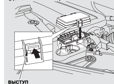
БЛОК ПРЕДОХРАНИТЕЛЕЙ В МОТОРНОМ ОТСЕКЕ (ДОПОЛНИТЕЛЬНЫЙ)
