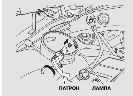
БОКОВОЙ ГАБАРИТНЫЙ ФОНАРЬ
