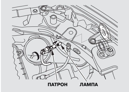
ГАБАРИТНЫЙ ФОНАРЬ
