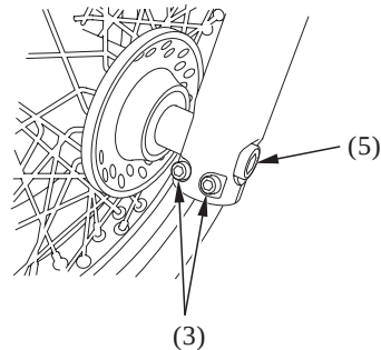
(5) Передняя ось
