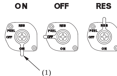
(1) Топливный кран
