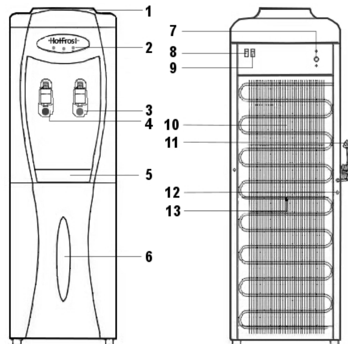
Рис.2 Схема аппарата V208...
