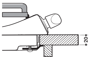
Монтаж крюка для опорных брусков H=30 мм
