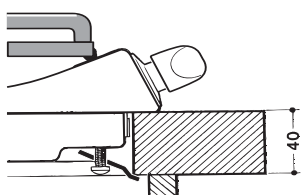
Монтаж крюка для опорных брусков H=40 мм
