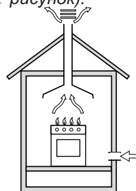
Прямое дымоудаление в атмосферу
