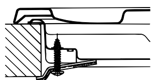
Монтаж крюка для опорных брусков H=40 мм Сзади
