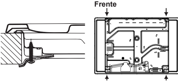
Posição do gancho para H=40mm
