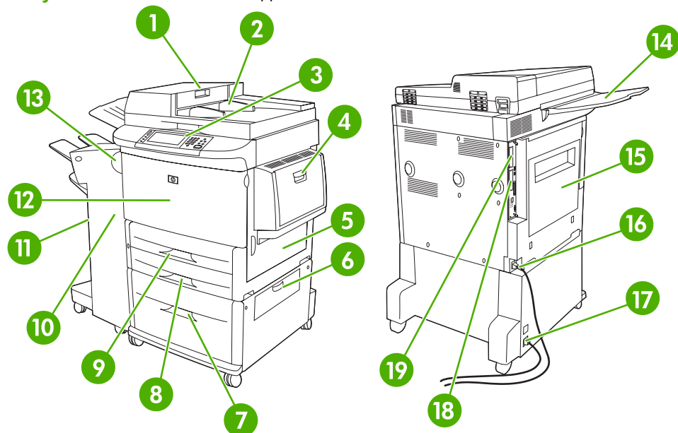
Рисунок 1-2 Компоненты изделия
