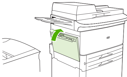
Рисунок 7-20 Изменение положения рычажков термоэлемента (4 из 4)
