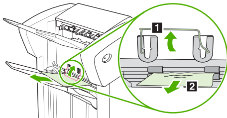
Рисунок 12-22 Удаление замятия в укладчике или шивателе/укладчике (3 из 7)
