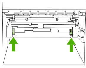
Рисунок 7-19 Изменение положения рычажков термоэлемента (3 из 4)
