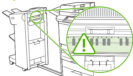
Рисунок 12-24 Удаление замятия в укладчике или шивателе/укладчике (5 из 7)
