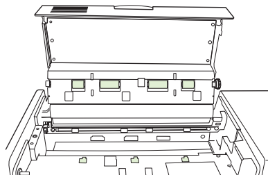
Рисунок 11-21 Очистка роликов устройства АПД (5 из 6)
