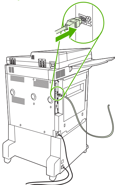
Рисунок 5-1 Подключение USB
