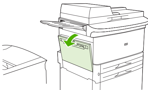
Рисунок 7-18 Изменение положения рычажков термозлемента (2 из 4)
