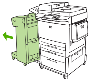
Рисунок 12-62 Устранение замятия за левой дверцей (1 из 4)
