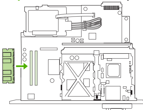
Рисунок 11-28 Установите модуль DIMM памяти DDR (6 из 8)
