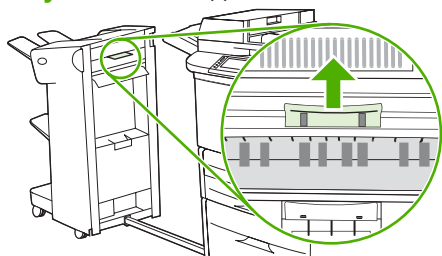
Рисунок 12-23 Удаление замятия в укладчике или шивателе/укладчике (4 из 7)
