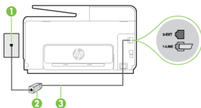
Рисунок Б-2 Вид принтера сзади
