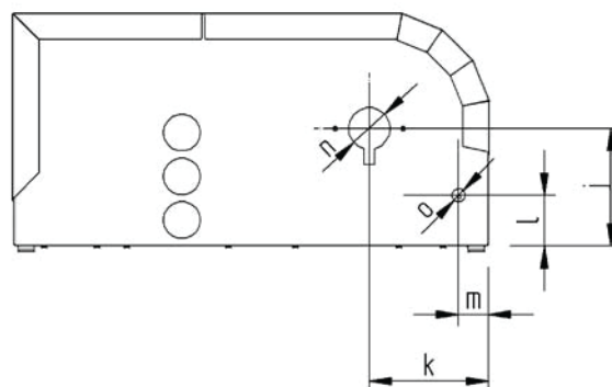
Вид сверху
