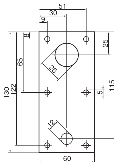
Фланец DN25 E-2604260
