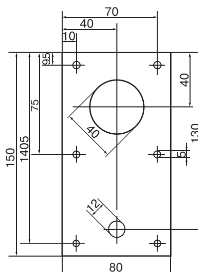
Фланец DN40 E-2604410
