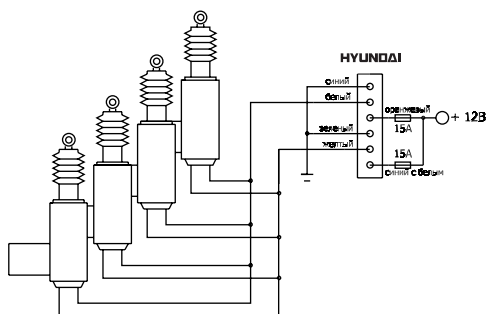
СХЕМА УПРАВЛЕНИЯ ДОПОЛНИТЕЛЬНЫМИ ЭЛЕКТРОПРОВОДАМИ
