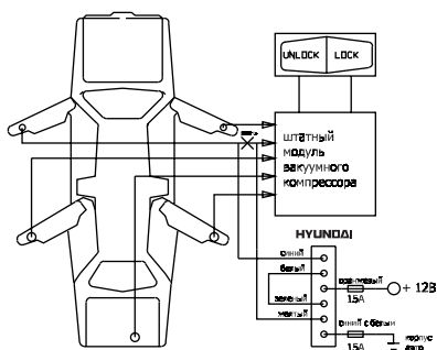
СХЕМА УПРАВЛЕНИЯ ВАКУУМНЫМИ СИСТЕМАМИ немецкого производства
