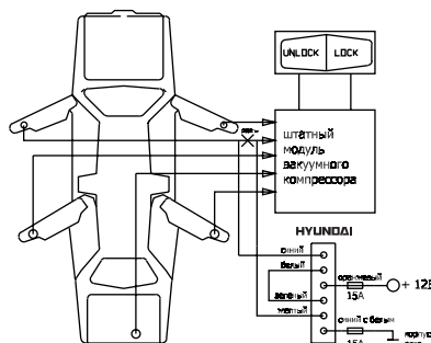
СХЕМА УПРАВЛЕНИЯ ВАКУУМНЫМИ СИСТЕМАМИ немецкого производства
