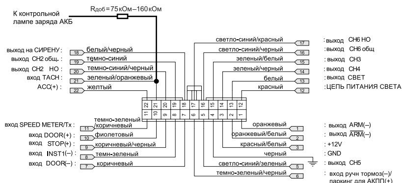
СХЕМА СОЕДИНЕНИЙ В РЕЖИМЕ АВТОЗАПУСКА БЕЗ ИСПОЛЬЗОВАНИЯ ТУРБОТАЙМЕРА
