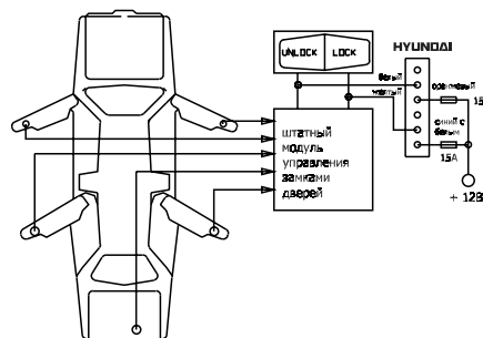
Положительный триггер (большинство легковых автомобилей американского производства)
