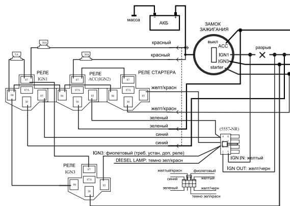
СХЕМА СОЕДИНЕНИЙ В РЕЖИМЕ АВТОЗАПУСКА С ИСПОЛЬЗОВАНИЕМ ТУРБОТАЙМЕРА И ДОПОЛНИТЕЛЬНОЙ ЛИНИИ ЗАЖИГАНИЯ IGN3
