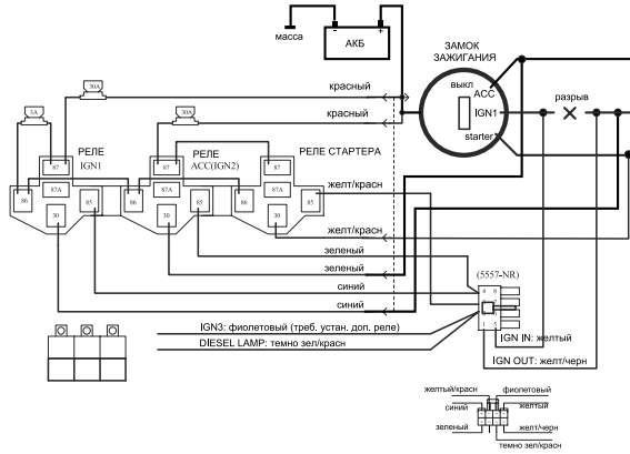
СХЕМА СОЕДИНЕНИЙ В РЕЖИМЕ АВТОЗАПУСКА С ИСПОЛЬЗОВАНИЕМ ТУРБОТАЙМЕРА И ЛИНИИ УПРАВЛЕНИЯ IGN3 АСС (вместо линии IGN2 АСС)
