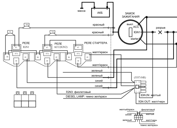
СХЕМА СОЕДИНЕНИЙ В РЕЖИМЕ АВТОЗАПУСКА С ИСПОЛЬЗОВАНИЕМ ТУРБОТАЙМЕРА И ДОПОЛНИТЕЛЬНОЙ ЛИНИИ ЗАЖИГАНИЯ IGN3
