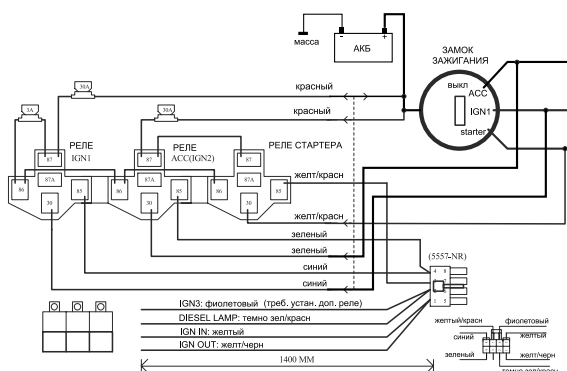
СХЕМА СОЕДИНЕНИЙ В РЕЖИМЕ АВТОЗАПУСКА БЕЗ ИСПОЛЬЗОВАНИЯ ТУРБОТАЙМЕРА
