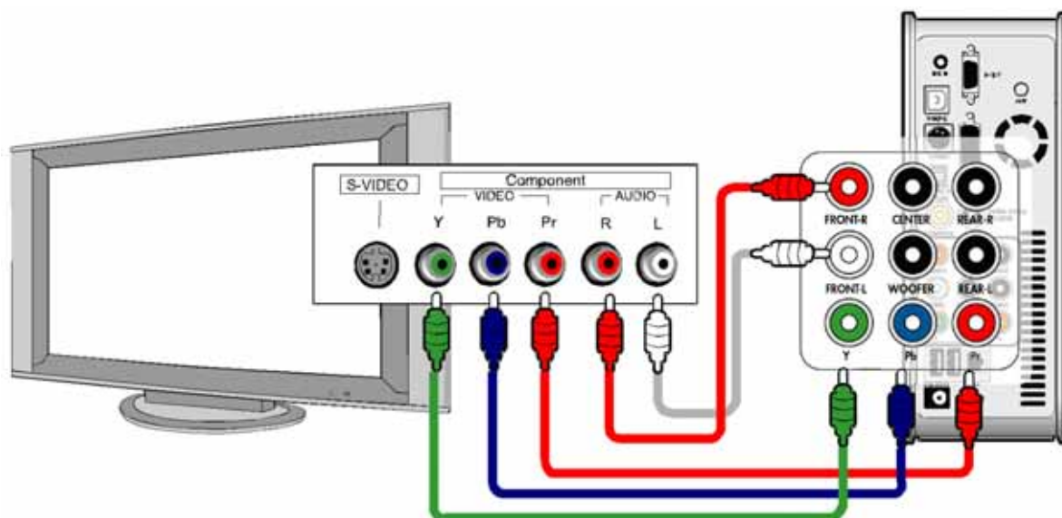
Соединение при помощи компонентного кабеля
