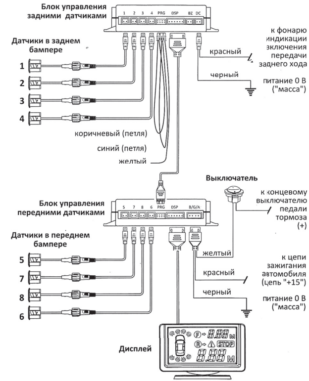
Схема установки Reverse Aid System - PT-218
