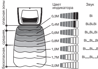
Рис. 5 Индикация опасности систем серии PS-LE
