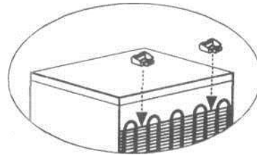
Рис.6 Схема установки задних упоров
