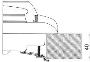
تركيب الخطافات بالنسبة للسطح الارتفاع=40 ملم
