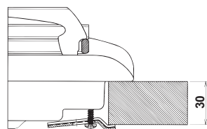
Position du crochet pour top H=30mm
