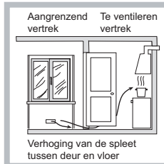
Voorbeelden ventilatie-opening voor verbrandingslucht
