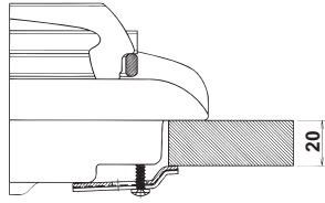
تركيب الخطافات بالنسبة للسطح الارتفاع=20 ملم
