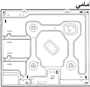
تركيب الخطافات بالنسبة للسطح الارتفاع=30 ملم
