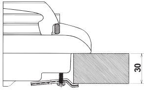
تركيب الخطافات بالنسبة للسطح الارتفاع=30 ملم
