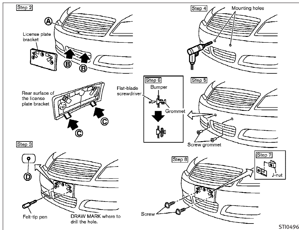
Sedan
