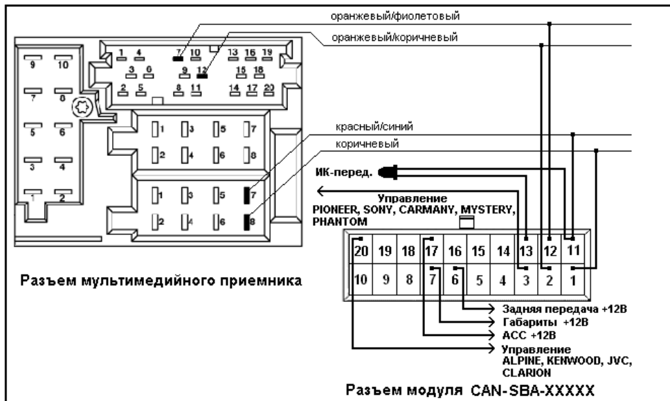
Рис. 2. Схема подключения модуля II
