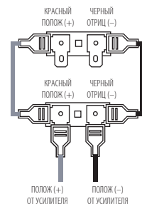
Рисунок 2. Параллельное подключение двух вуферов к усилителю (2 Ома)
