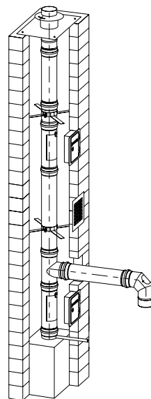
Рис. 3: стандартное устройство
