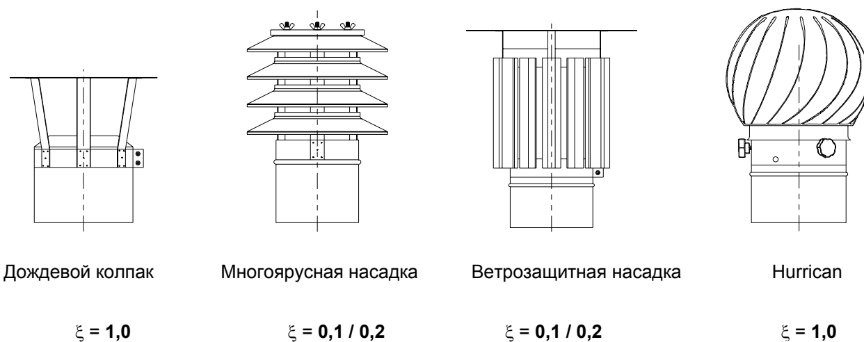
Рис. 6: Насадки
