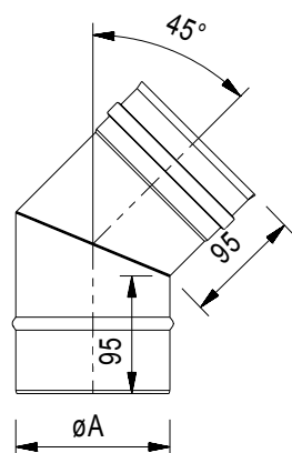
fu 19 Колено 45°
