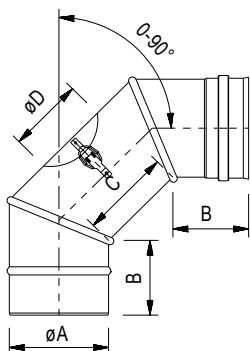
fu 102 Колено регулируемое 0-90° с лючком ревизии
