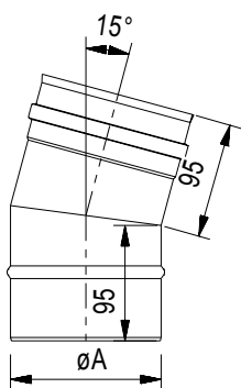
fu 17 Колено 15°
