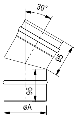
fu 18 Колено 30°
