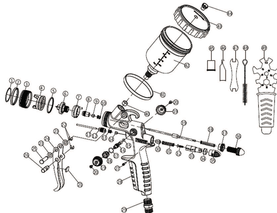
Рис. 5. Схема краскораспылителя модели КРП - 1,0/0,12ВБ ПРОФИ:
