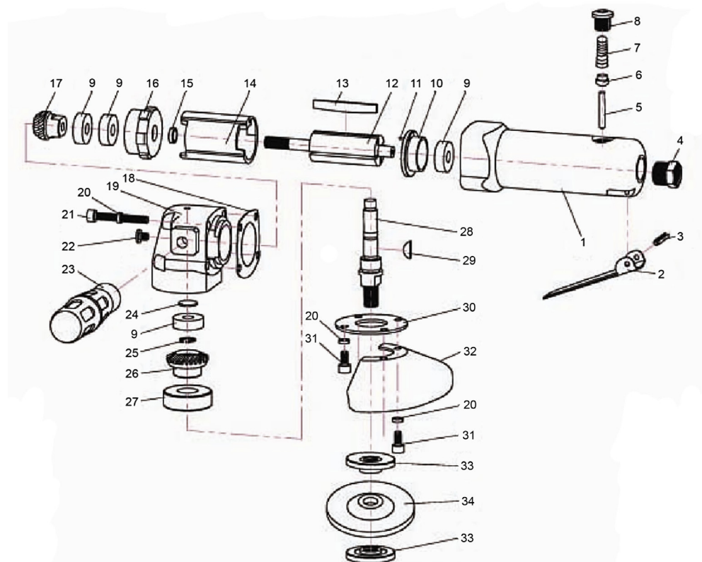
Рис. 3. Схема шлифмашины модели ПМШУ - 6,3/ 125
