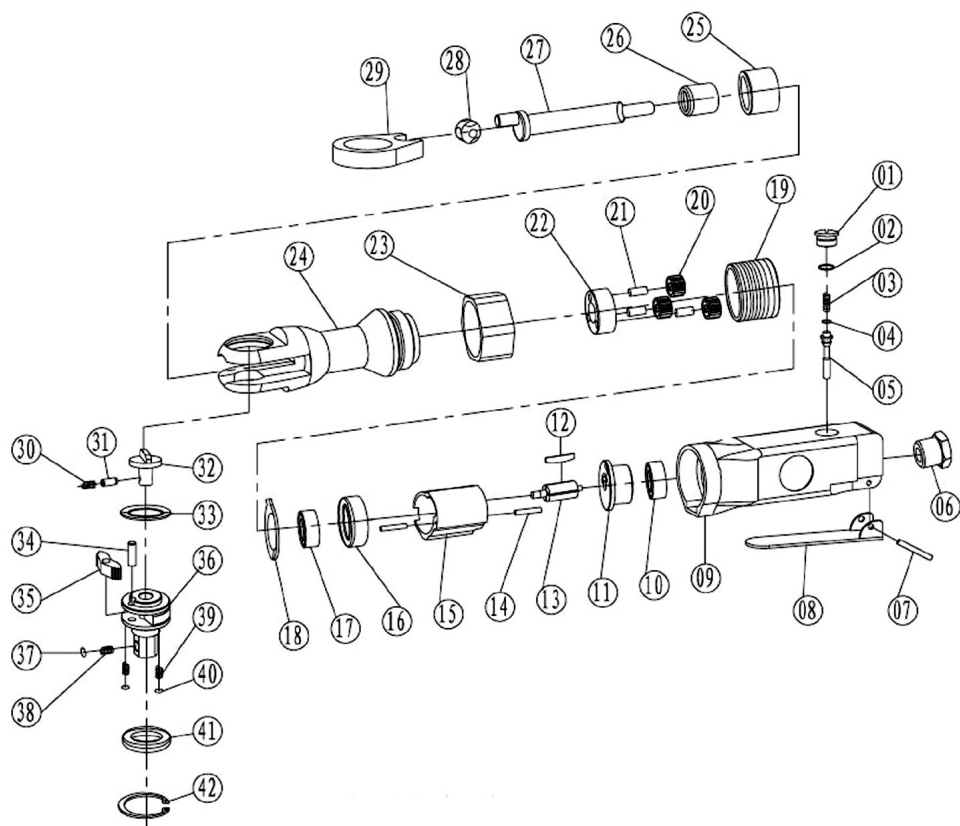
Рис. 3. Схема трещётки модели ПТ - 13/70
